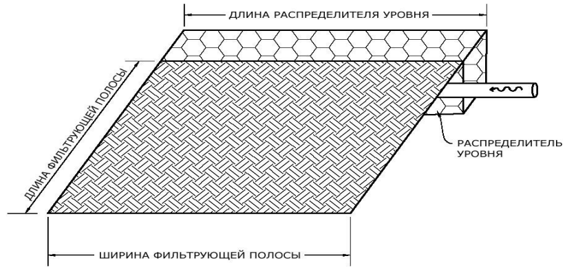
Рисунок 8 – Типовой профиль фильтрующей полосы
