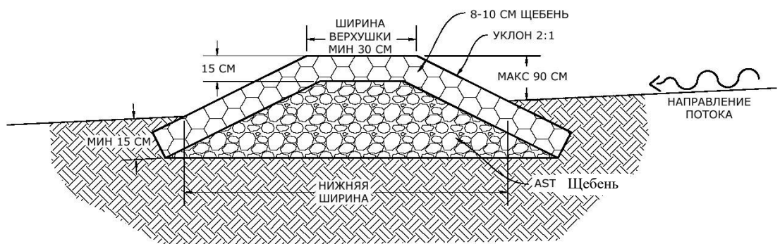
Рисунок 10 – Типовой профиль бермы перед фильтрующей полосой
