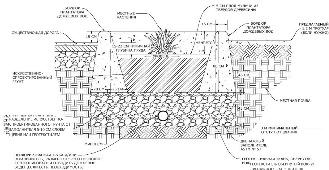
Рисунок 31 – Типовой профиль плантатора
