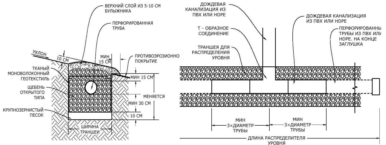
Рисунок 9 – Типовой профиль траншеи распределителя уровня
